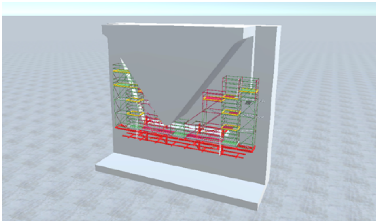
3D schets van het project waar Mark aan werkt
